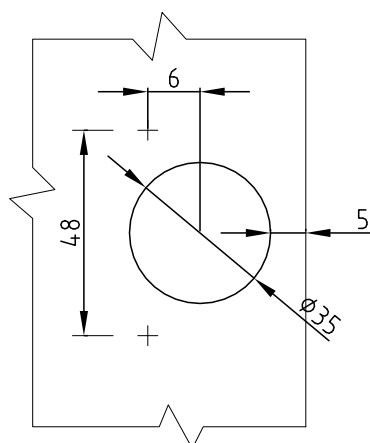
门板
