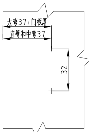
侧板
